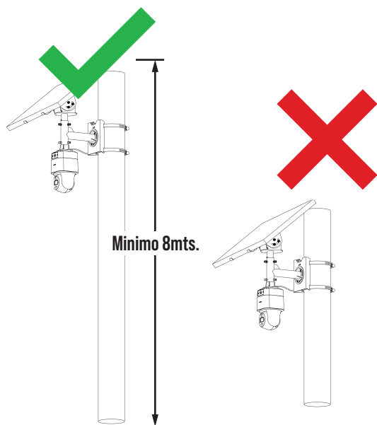
1. Sistema de monitoreo autónomo que no se encuentra a la altura adecuada.
