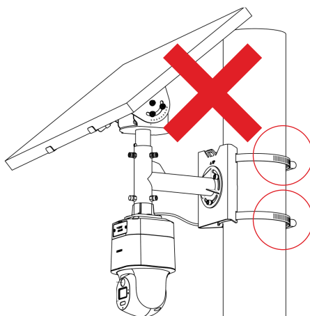
4. Sistema de monitoreo autónomo instalado en un poste o caño de poco espesor sin el debido ajuste de las abrazaderas.
